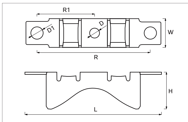
Držák na sloup "LONG BRIDGE", pro 2 - 3 šrouby
