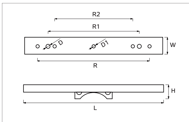
Držák na sloup "EXTREM BRIDGE"
